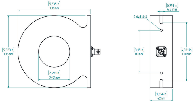
Abbildung 4 - PMK LILCO®-Serie 58: Mechanische Abmessungen
