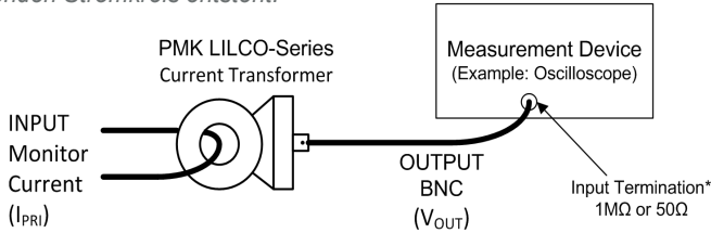
Abbildung 2 - Standard-Anschluss an den zu prüfenden Stromkreis Siehe Auswahltable für BNC-Ausgangsanschlüsse
