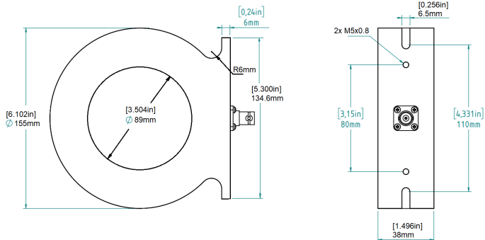
Abbildung 5 - PMK LILCO®-Serie 89: Mechanische Abmessungen
