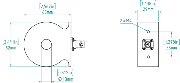
Abbildung 3 - PMK LILCO®-Serie 13: Mechanische Abmessungen
