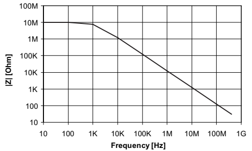
Typical input impedance PKT520A-RO
